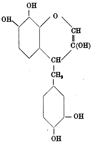
Hämatoxylin
